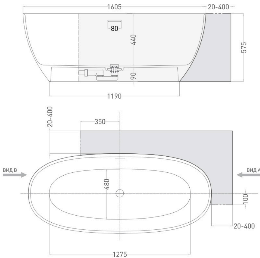
Пример установки ванны с угловой правой модификацией.
